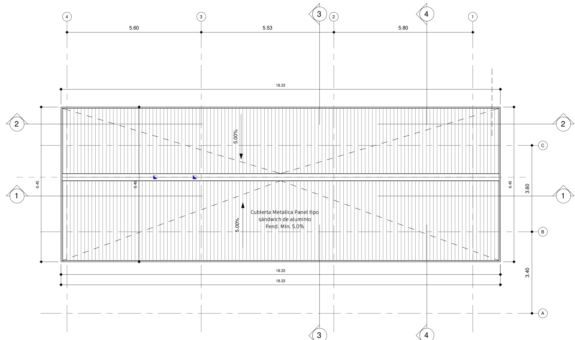
3 Casa 1 Cubierta 1:75
