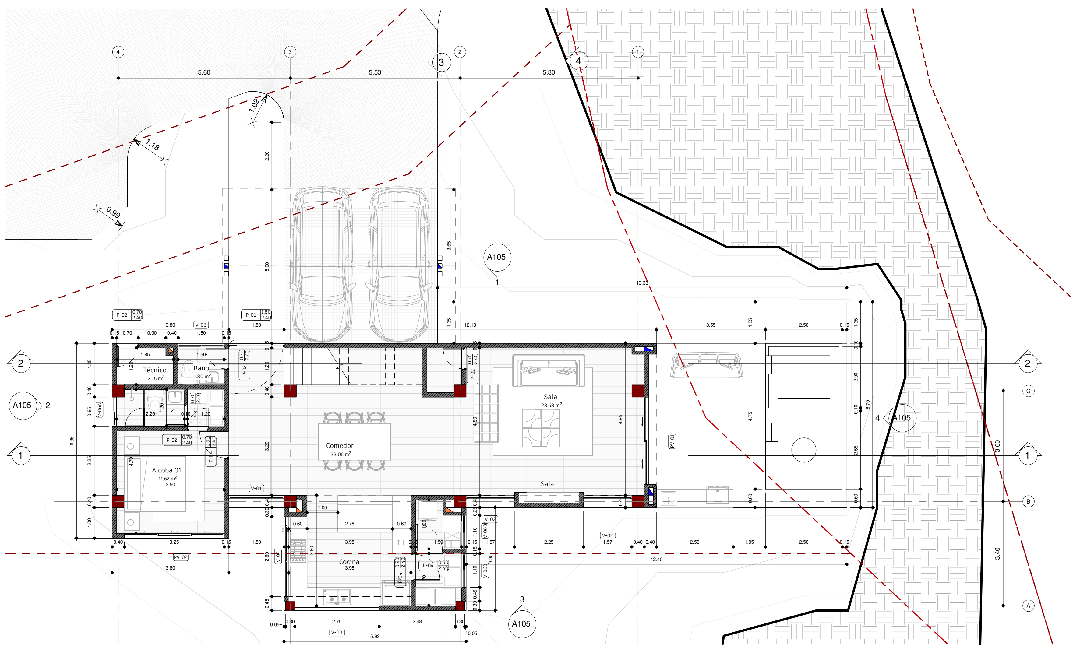
1 Casa 1 P1 1:75
