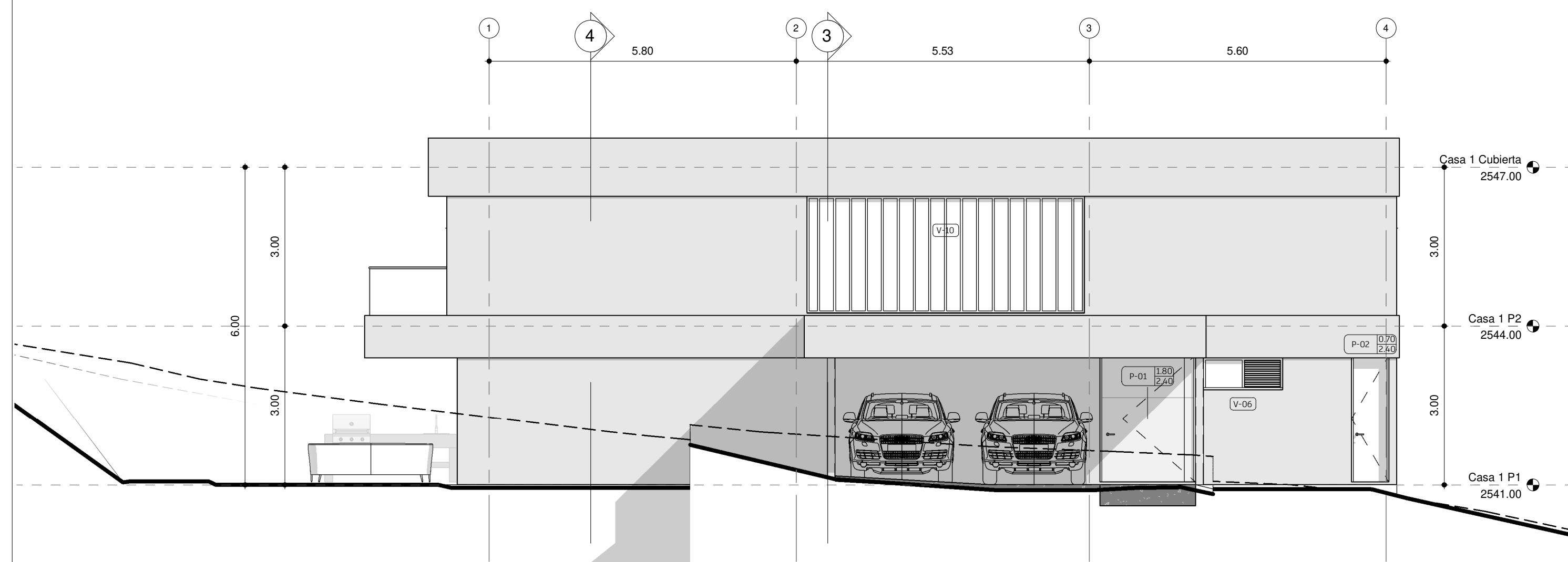
1 C1-FAC 1 1:75
